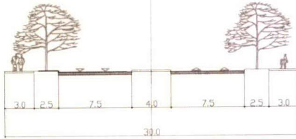
presjek 2-2
