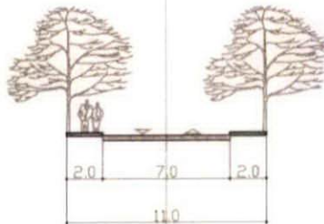
presjek 4-4
