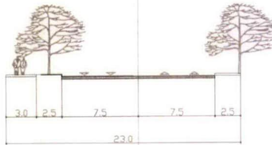
presjek 2-2
